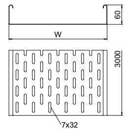
Abmessungen
