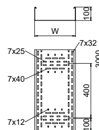
Abmessungen
